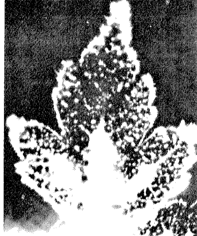
شكل ( ١٠ ب ) ورقة نبات تشع شحناتها الكهربائية على الفيلم الحساس فتبدو بهذه الهالة الفريية .
